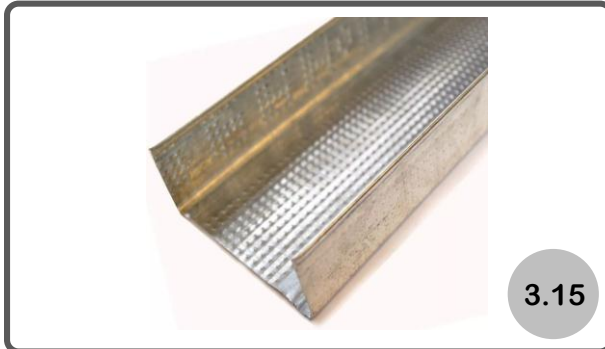
Solera 70 mm Esp. 0,5 Largo 3 m
