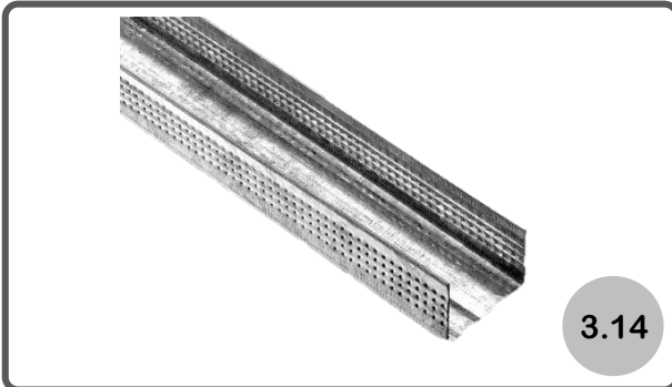
Solera 35 mm Esp. 0,5 Largo 3 m
