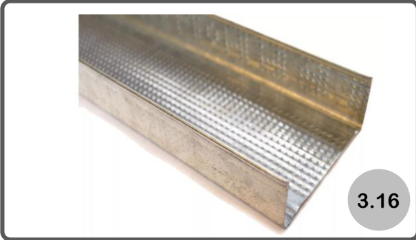
Solera 100 mm Esp. 0,5 Largo 3 m
